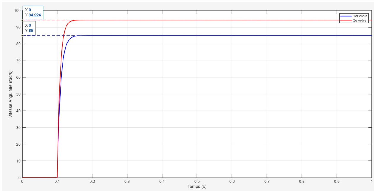
FIGURE 3 : Comparaison entre le modèle du 1 er ordre identifié et le produit G_{\text{elec}}(s) \cdot G_{\text{mot}}(s)
