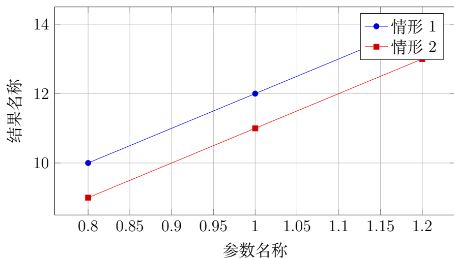
图 4 敏感性分析图
