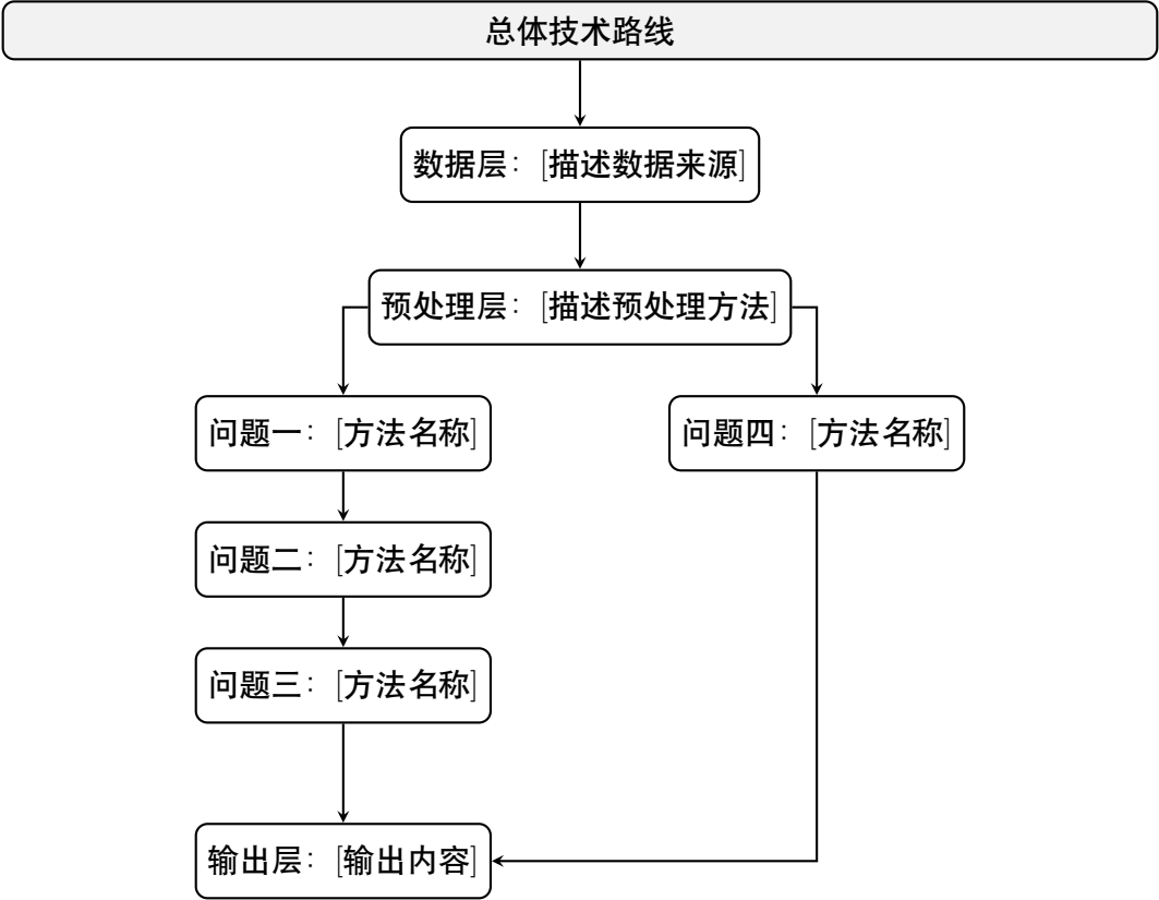
图 1 总体技术路线流程图
