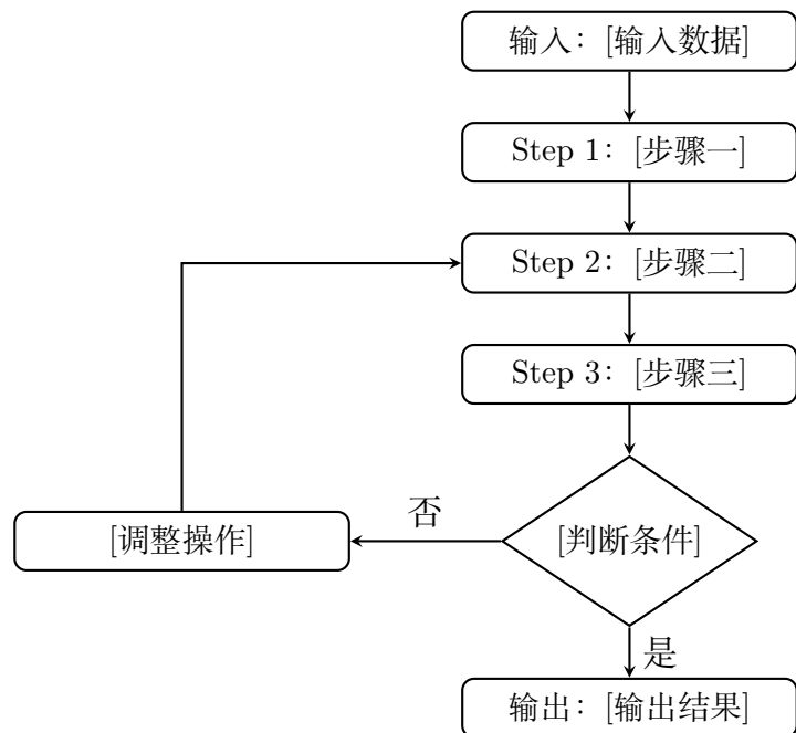
图 5 单品级组合优化求解流程图
