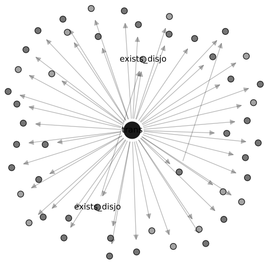
out_degree (high) trans (val=1538)
