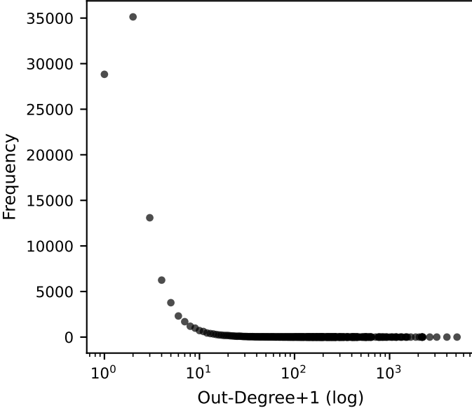
out_degree (high)
