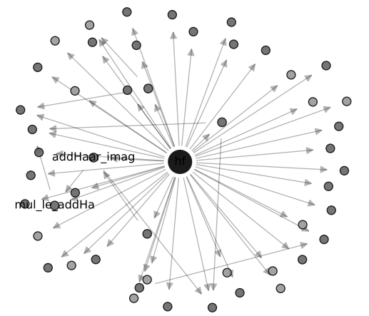
out_degree (high)
