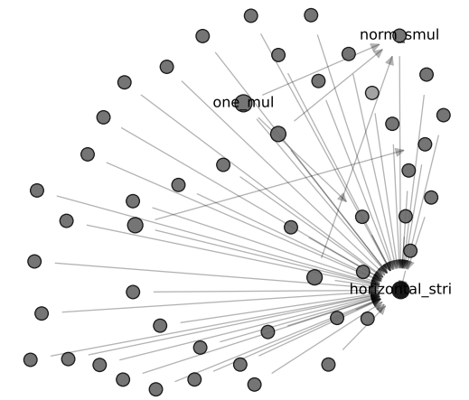
in_degree (high)
