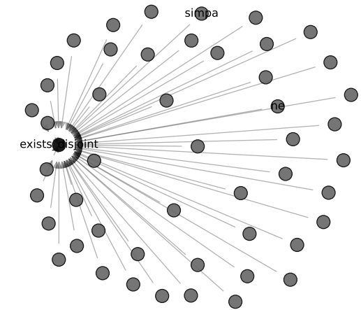
in_degree (high)
