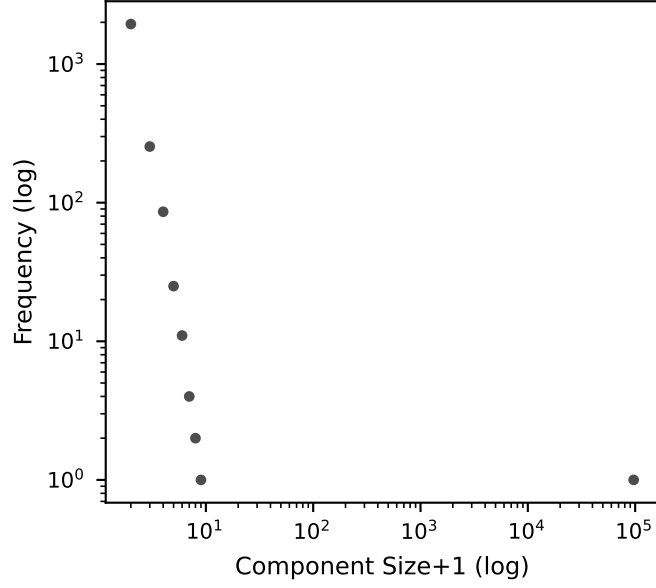
out_degree (high)
