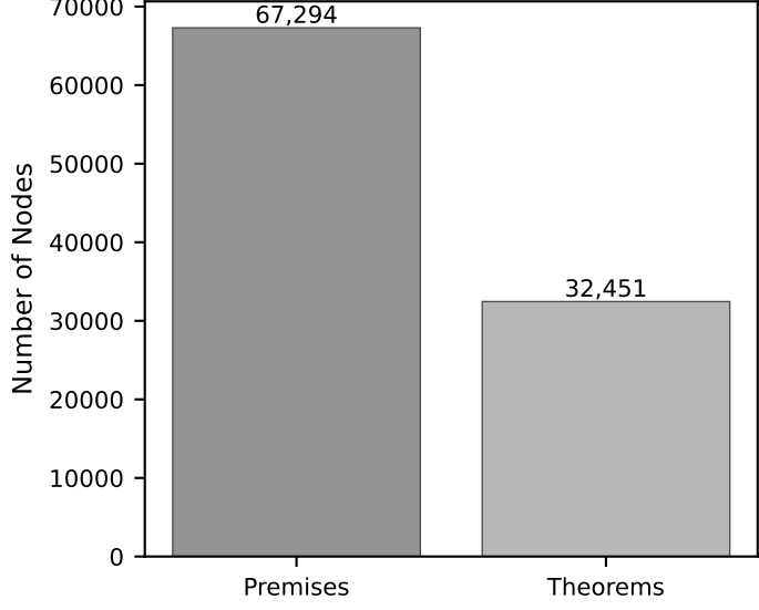
in_degree (high)
