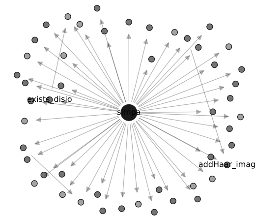
out_degree (high)
