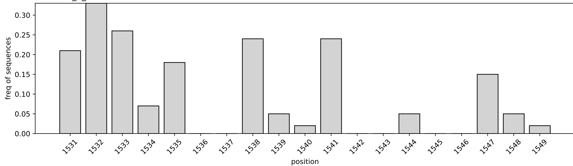
varVAMP_2_RIGHT
