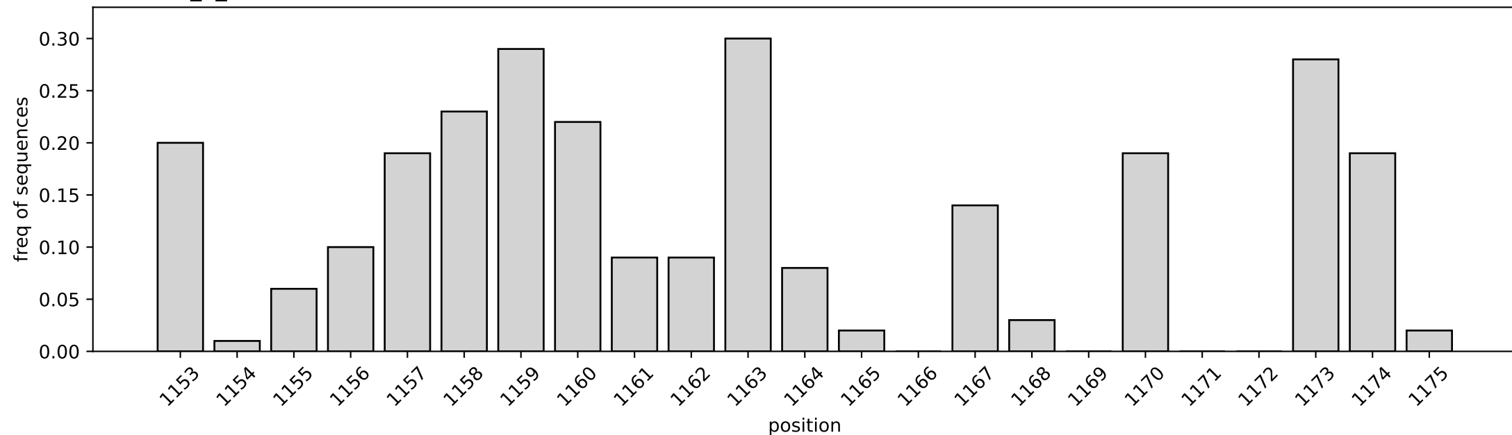
varVAMP_2_LEFT
