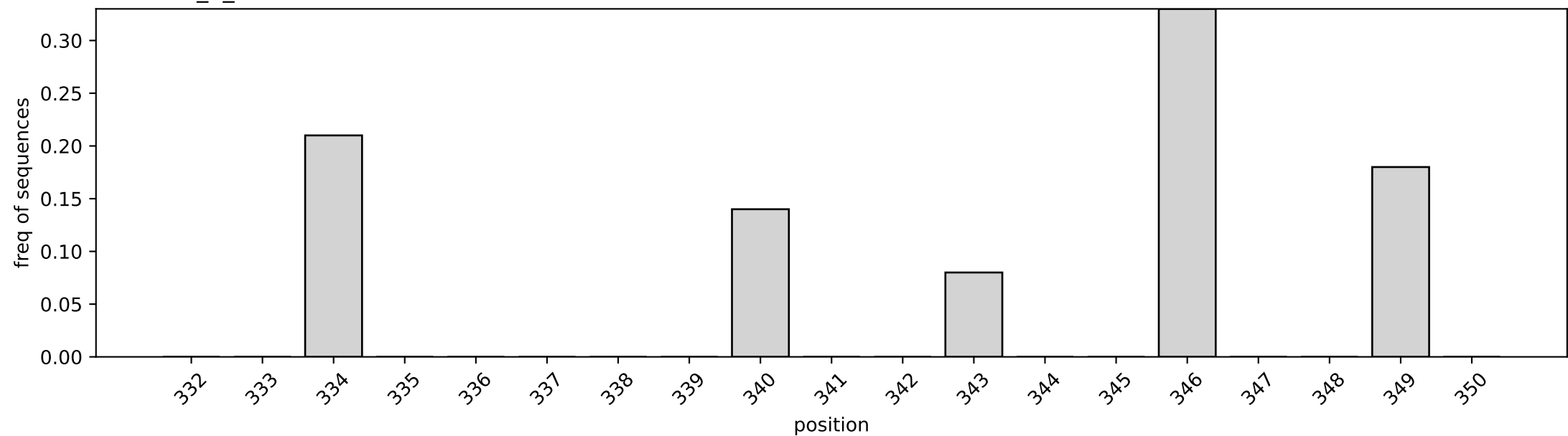
varVAMP_0_RIGHT
