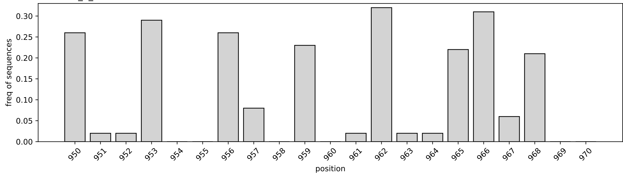
varVAMP_1_RIGHT
