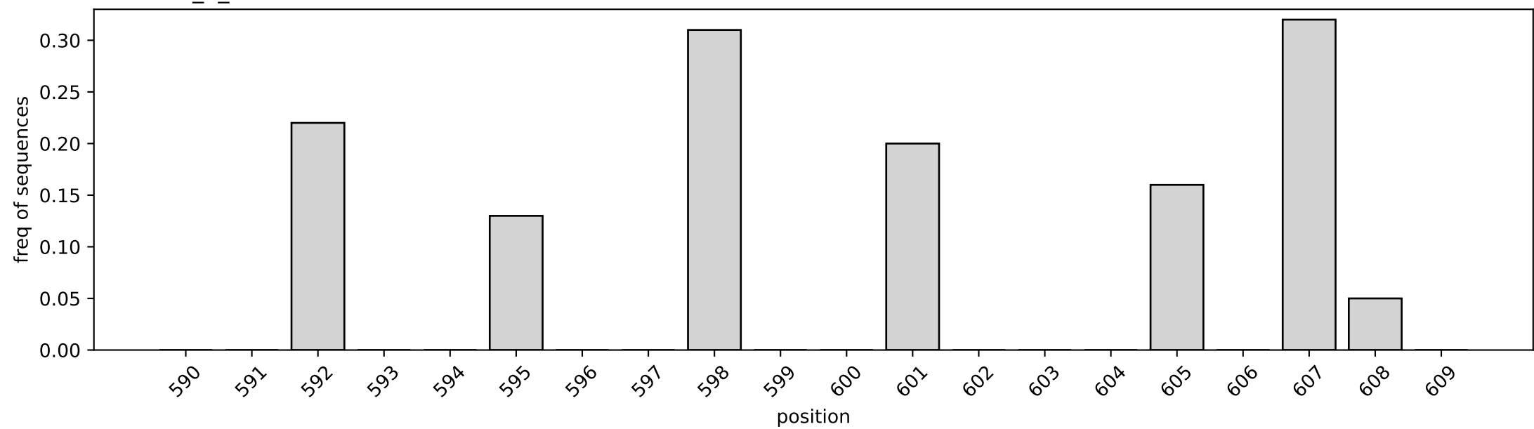
varVAMP_1_LEFT
