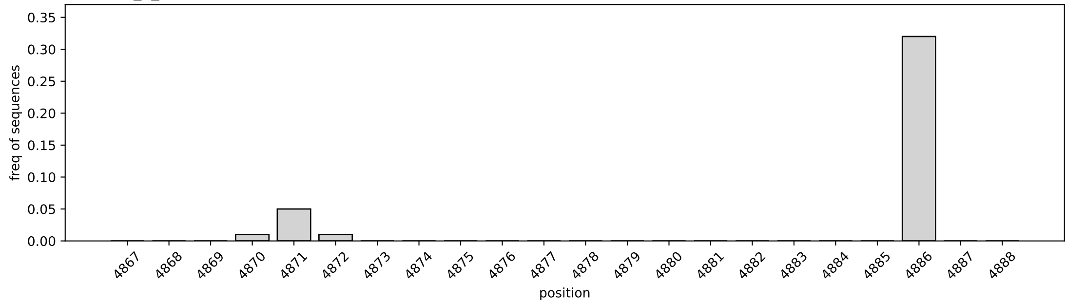
varVAMP_0_RIGHT
