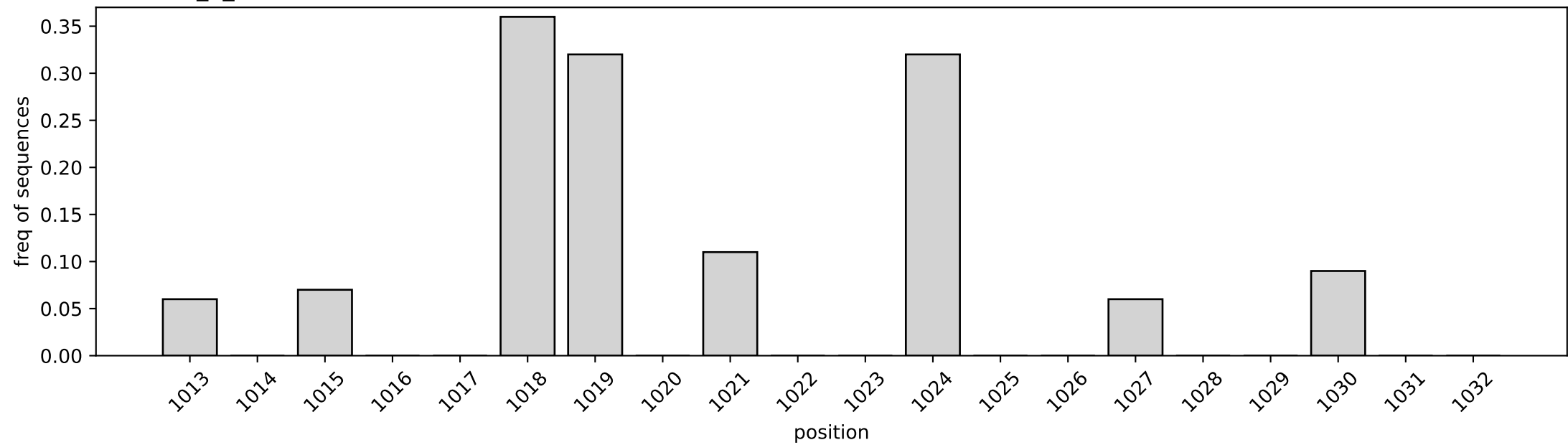
varVAMP_1_LEFT
