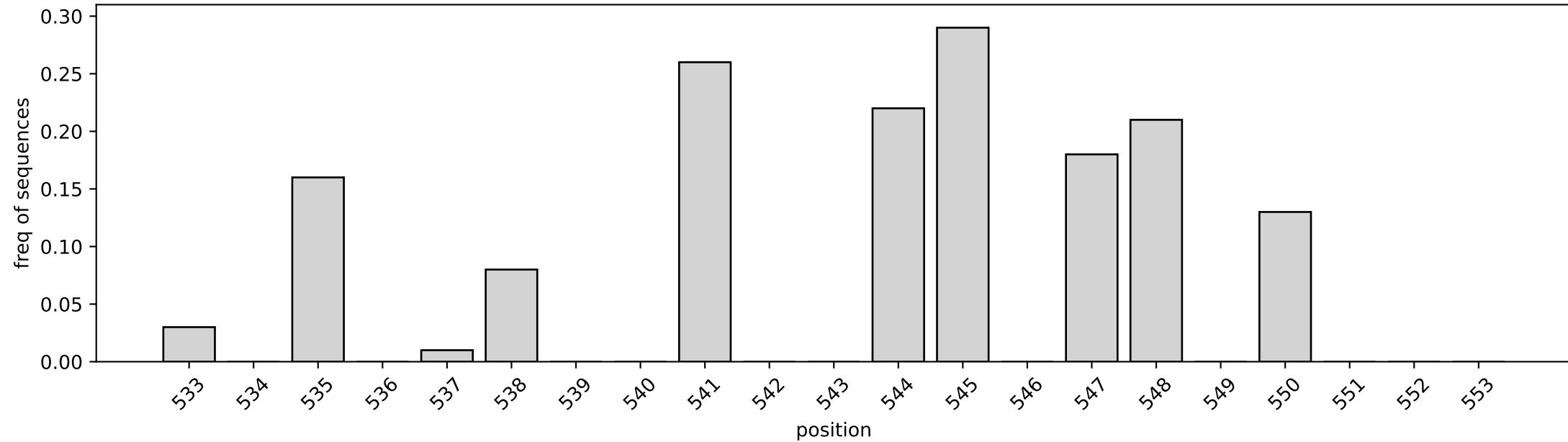
varVAMP_2_LEFT
