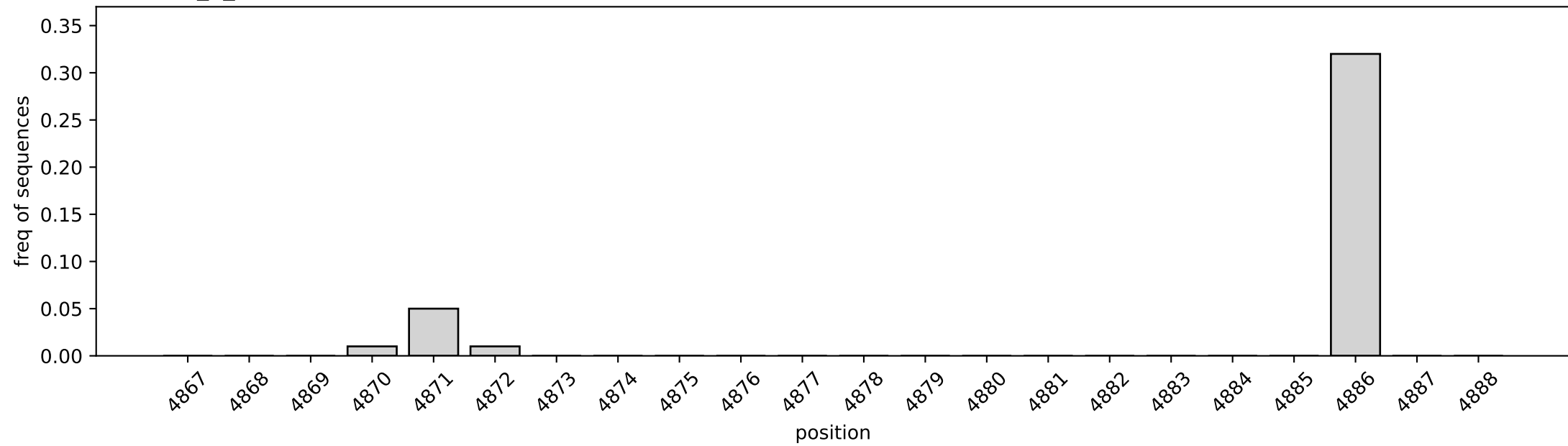
varVAMP_0_RIGHT
