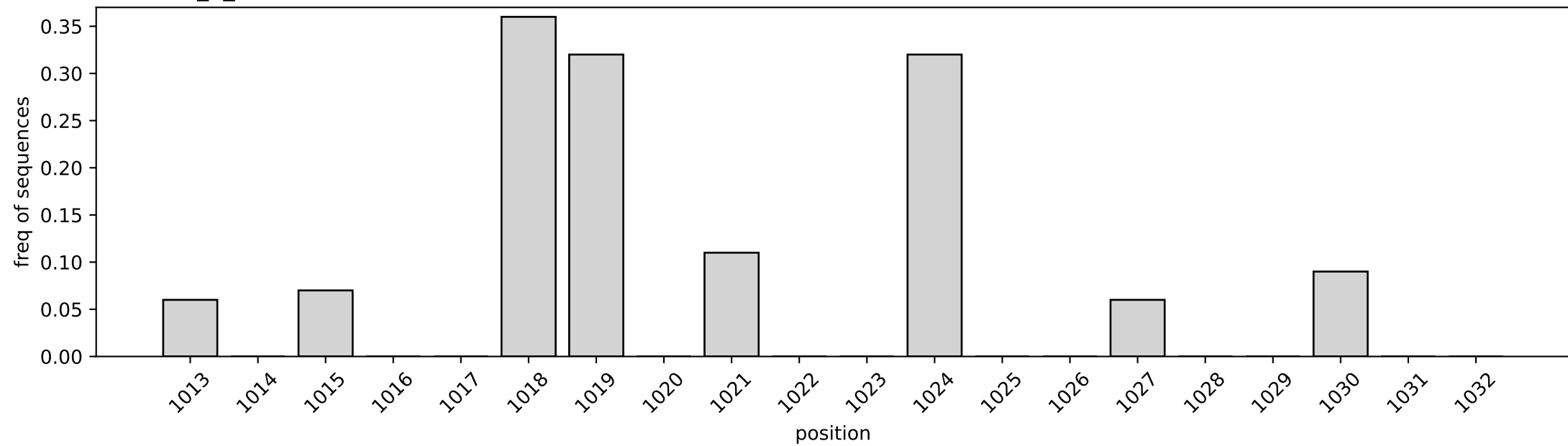
varVAMP_1_LEFT
