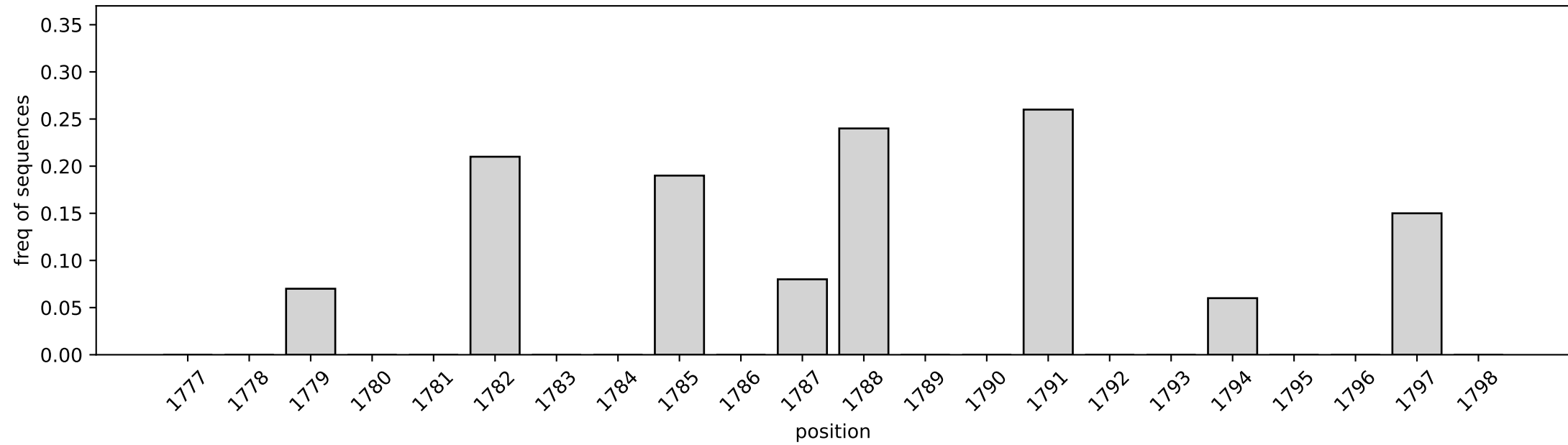
varVAMP_1_RIGHT
