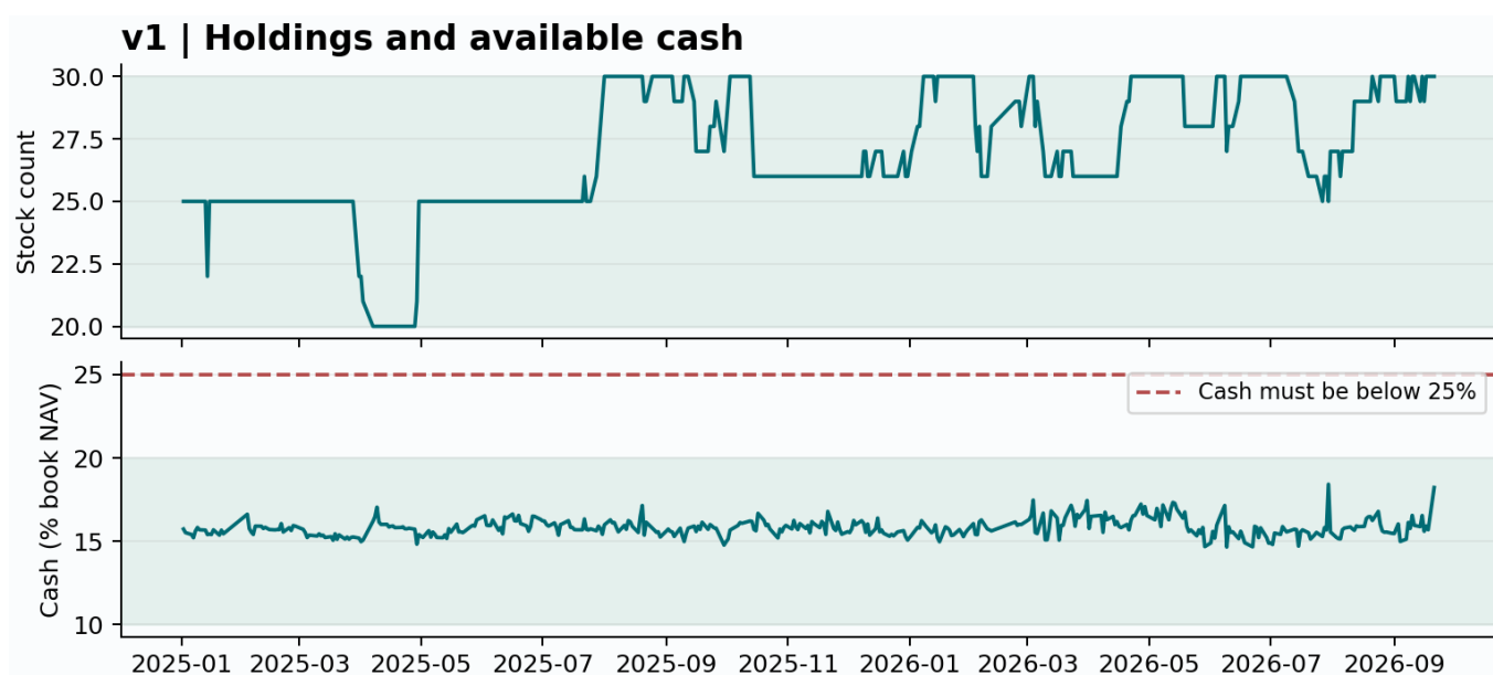
實際持股檔數與現金比例
