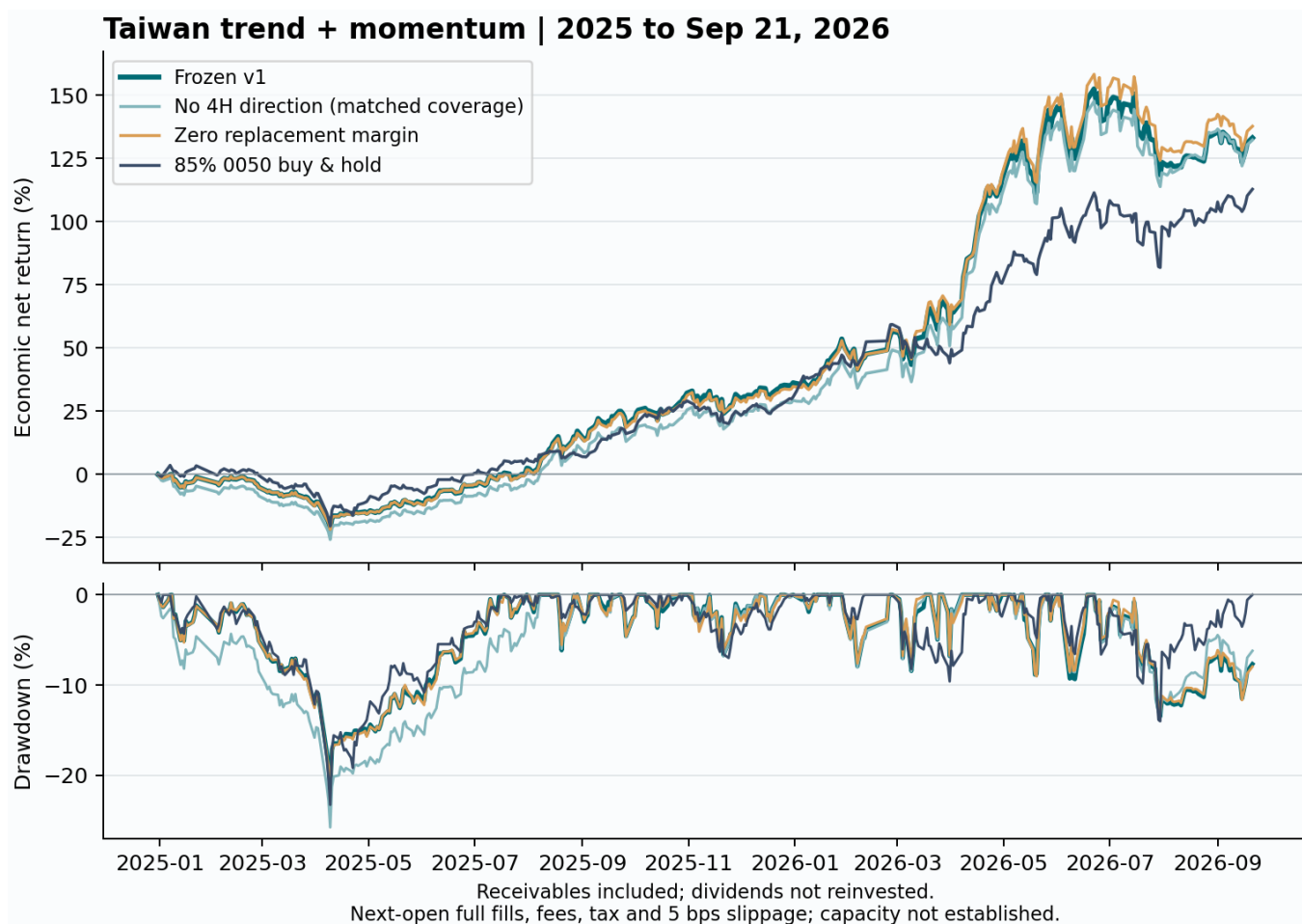
連續投組的經濟報酬與回撤
