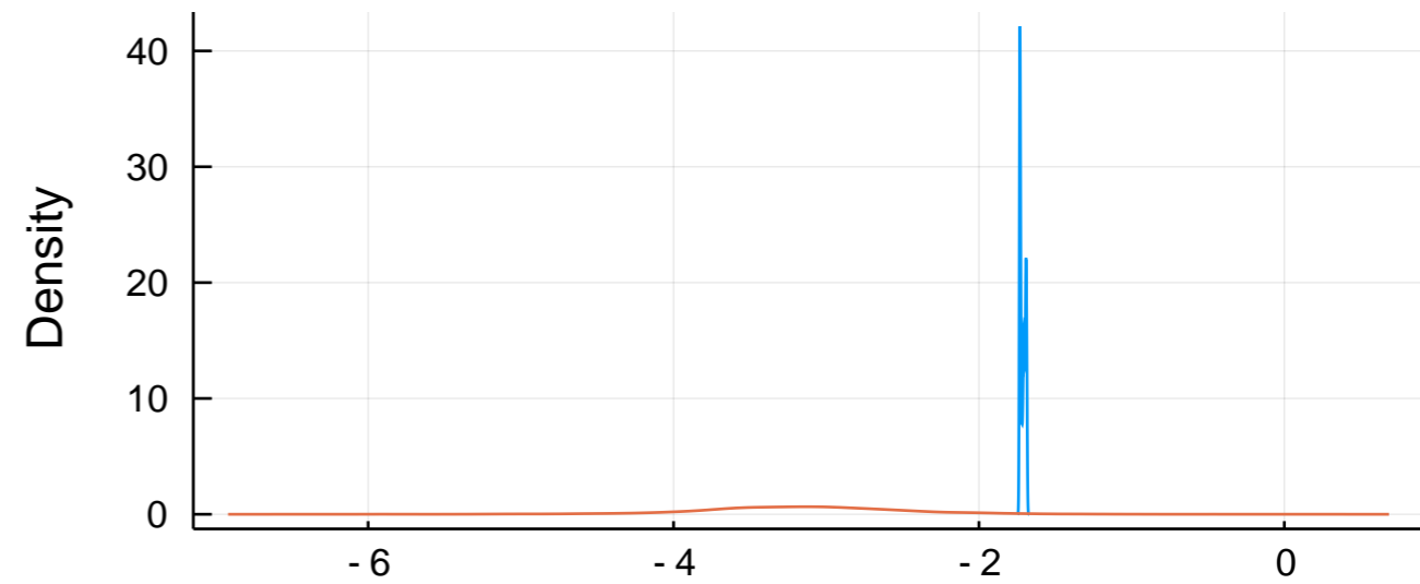
muh.1
