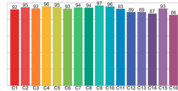
TM-30: 92,9
