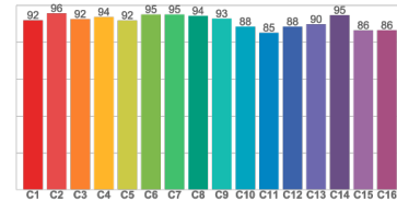
TM-30: 91,2
