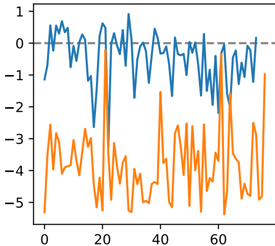
Session 1, CDdotprod 0.482
