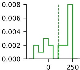
TDnet
