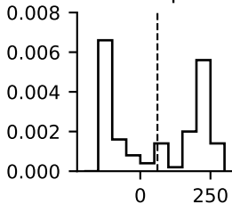
TDintp0
