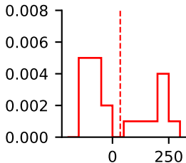
A2C
