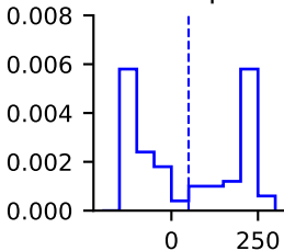
TDintp1
