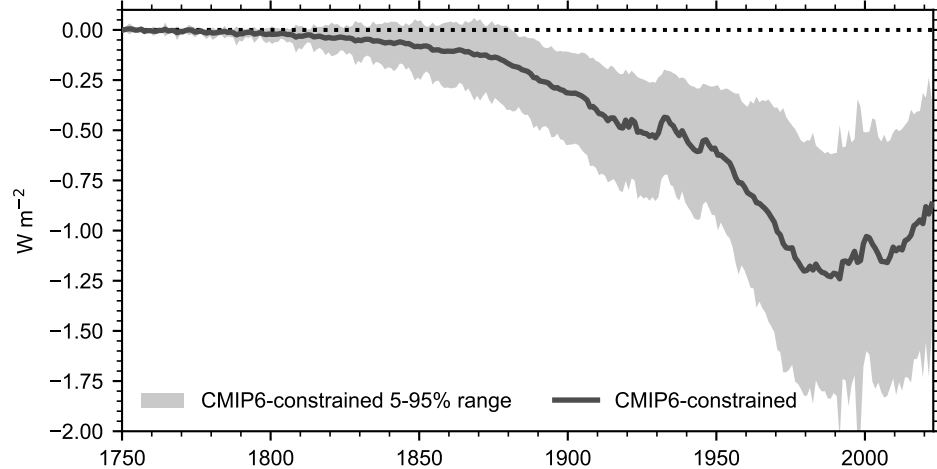
(c) Total aerosol ERF
