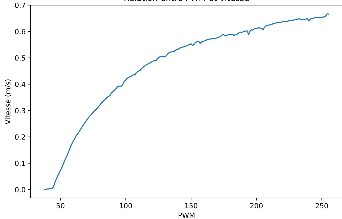
Relation entre PWM et vitesse
