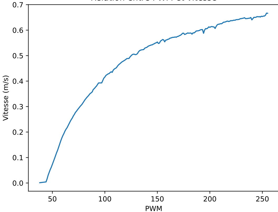
Relation entre PWM et vitesse
