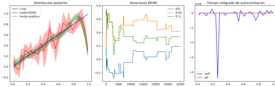
Figura 0.1: Resultados de los puntos 3, 4 y 5. Izquierda: distribución posterior con bandas de incertidumbre. Centro: cadenas MCMC para tres parámetros. Derecha: tiempo integrado de autocorrelación (IAT) y tamaño efectivo de muestra (neff) por parámetro.
