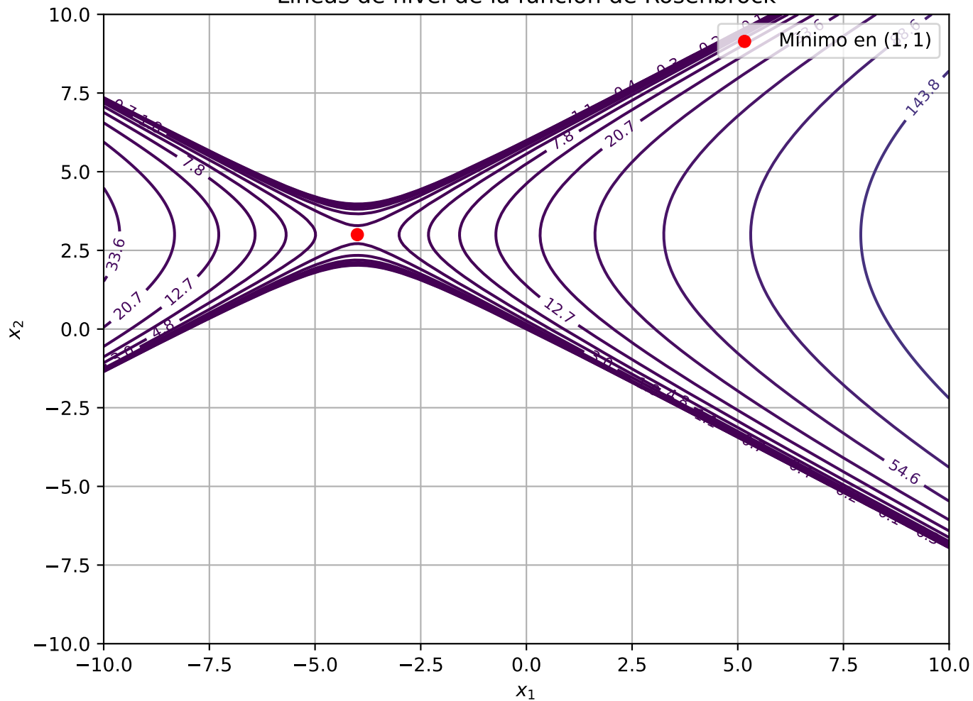
Líneas de nivel de la función de Rosenbrock
