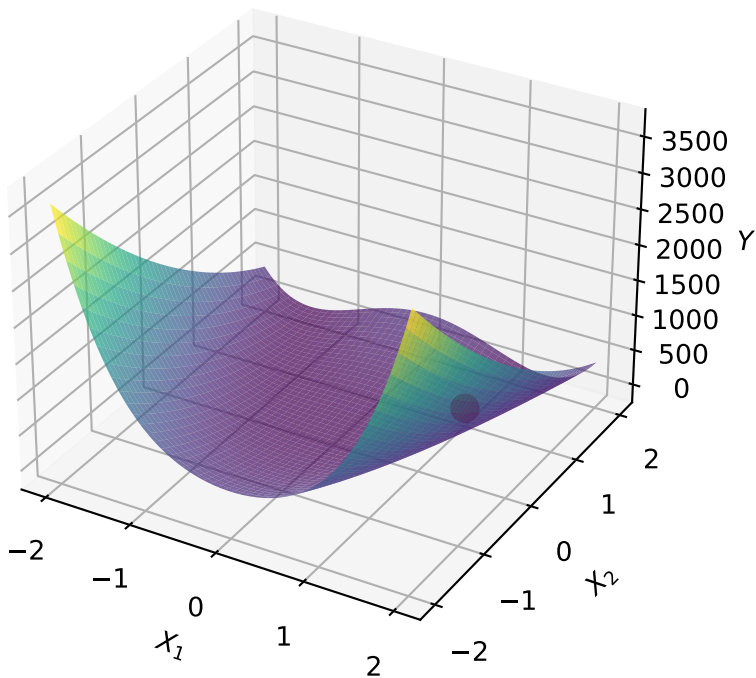
Gráfica de la función F(x_1, x_2) .
