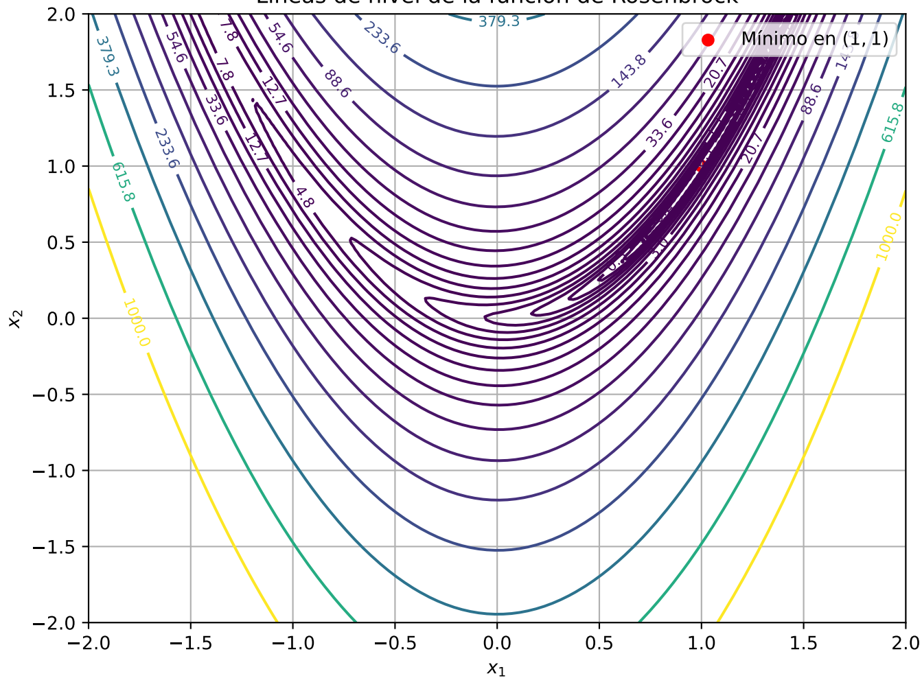
Líneas de nivel de la función de Rosenbrock
