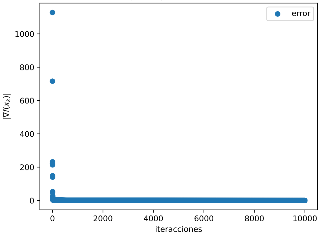
Gráfica |\nabla f(x_k)| de Rosenbrock 200D
