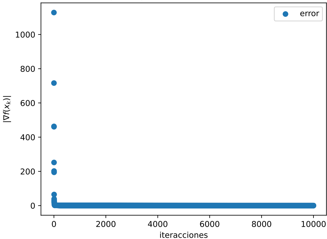
Gráfica |\nabla f(x_k)| de Rosenbrock 200D \delta = 0.001
