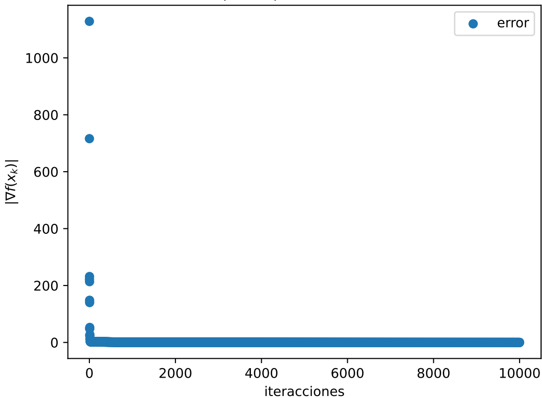
Gráfica |\nabla f(x_k)| de Rosenbrock 600D
