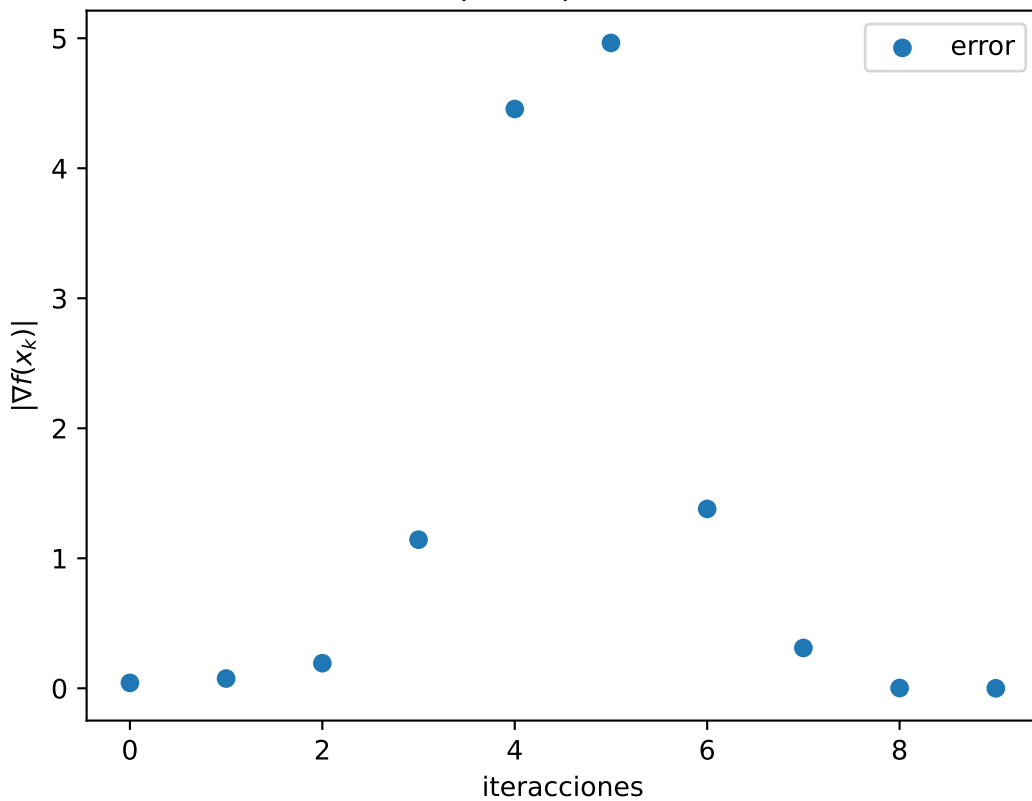
Gráfica |\nabla f(x_k)| de Hartmann
