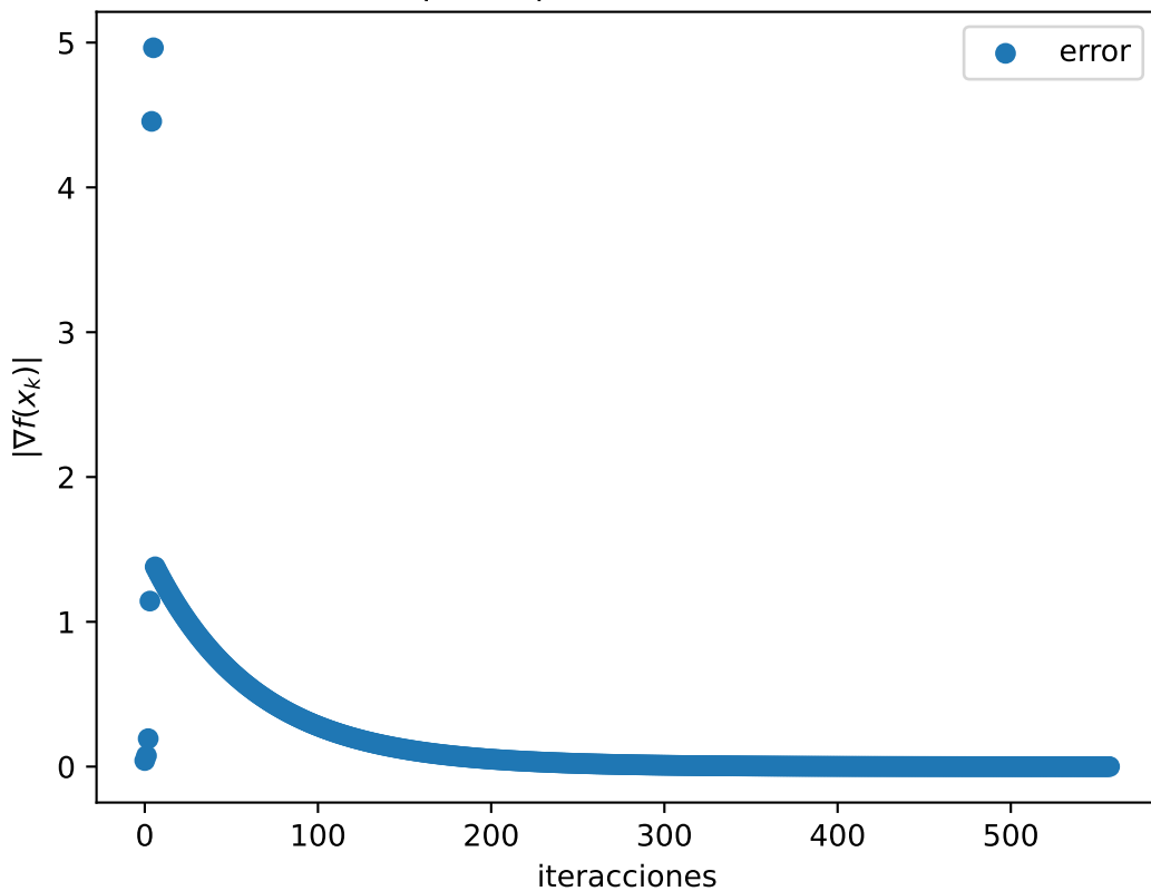
Gráfica |\nabla f(x_k)| de Hartmann \delta = 0.001
