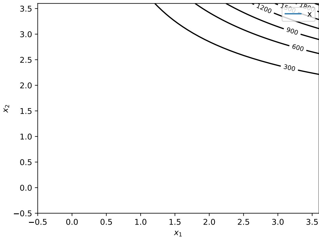
Gráfica de Beale \delta = 10.0
