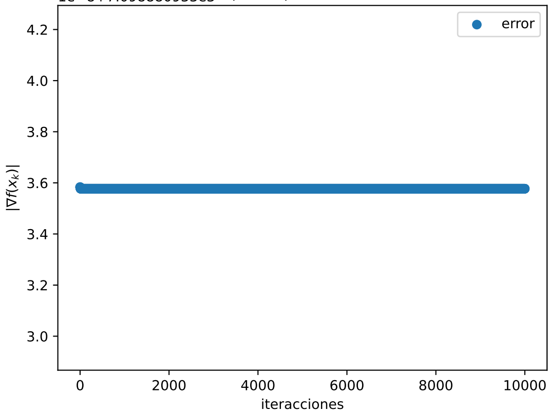
Gráfica |\nabla f(x_k)| de Beale \delta = 10.0
