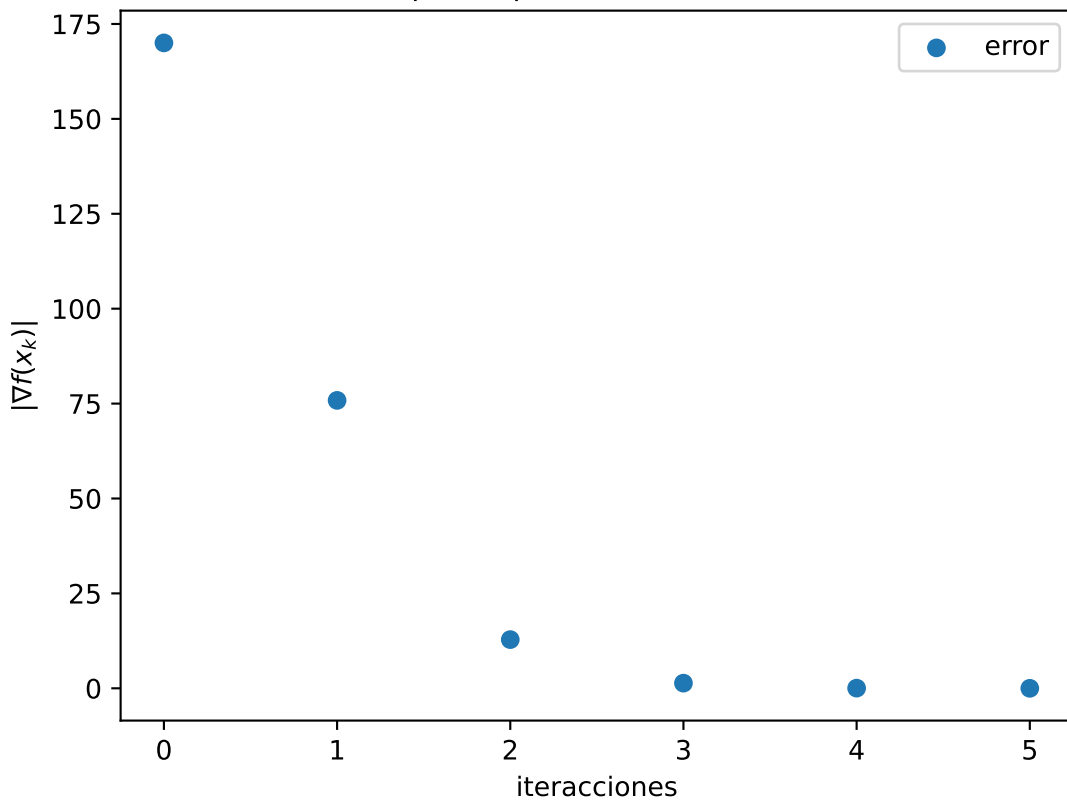
Gráfica |\nabla f(x_k)| de Himmelbau \delta = 10.0
