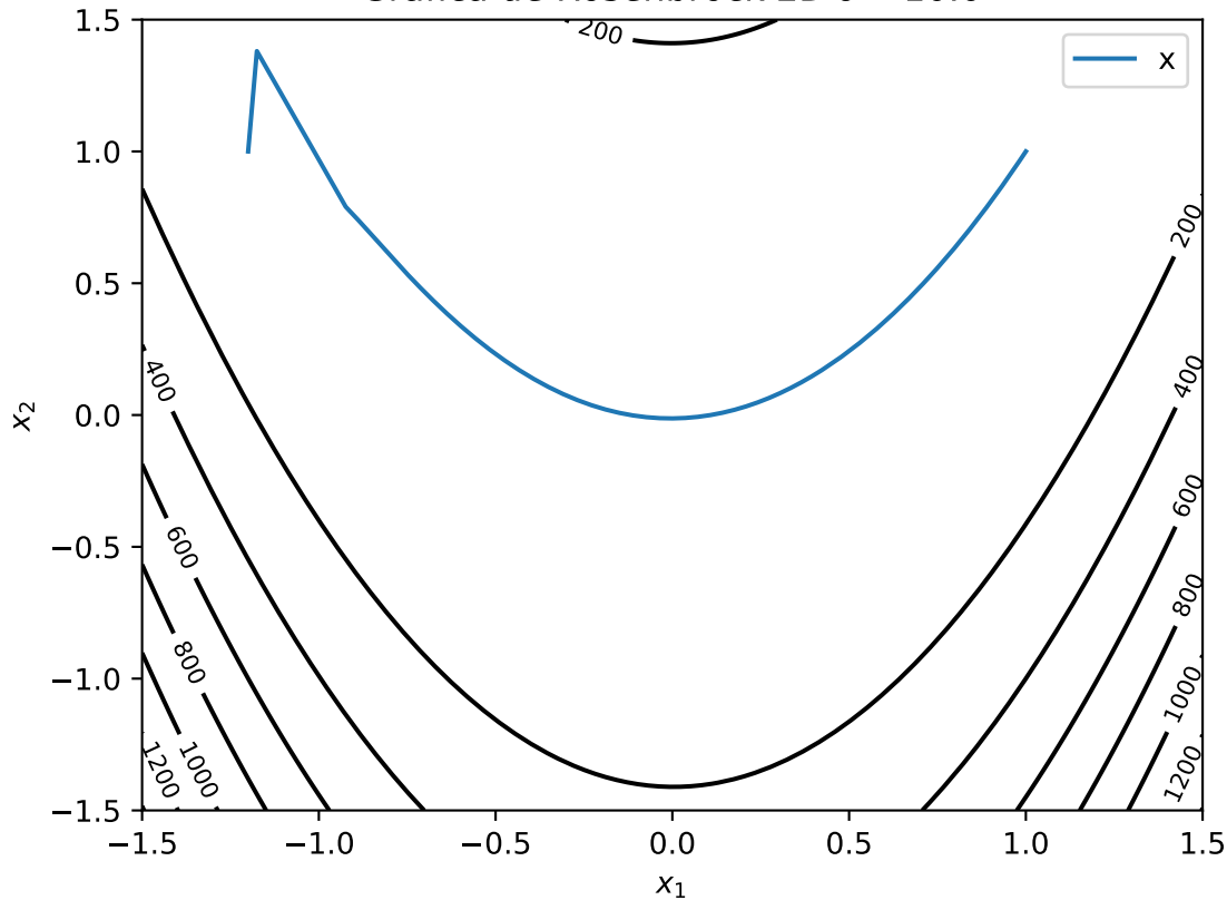
Gráfica de Rosenbrock 2D \delta = 10.0
