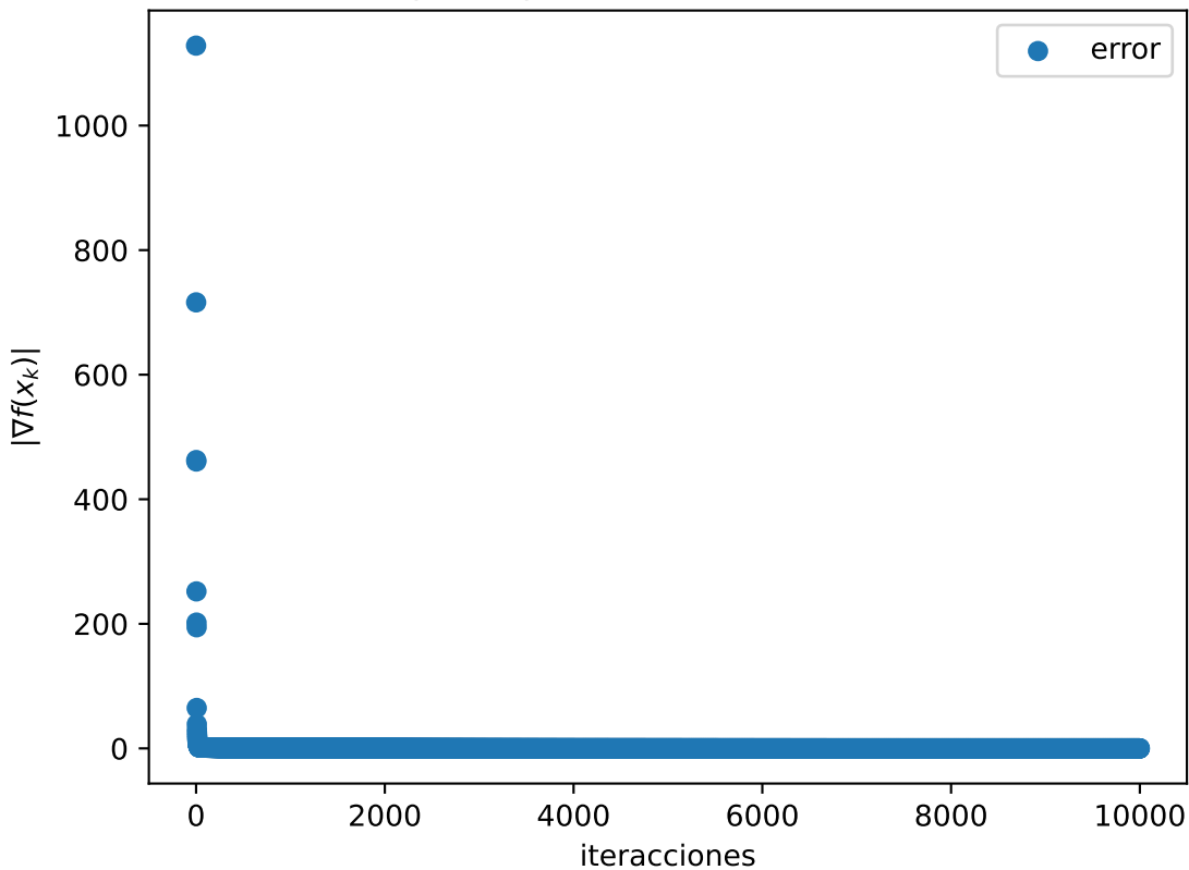
Gráfica |\nabla f(x_k)| de Rosenbrock 600D \delta = 10.0
