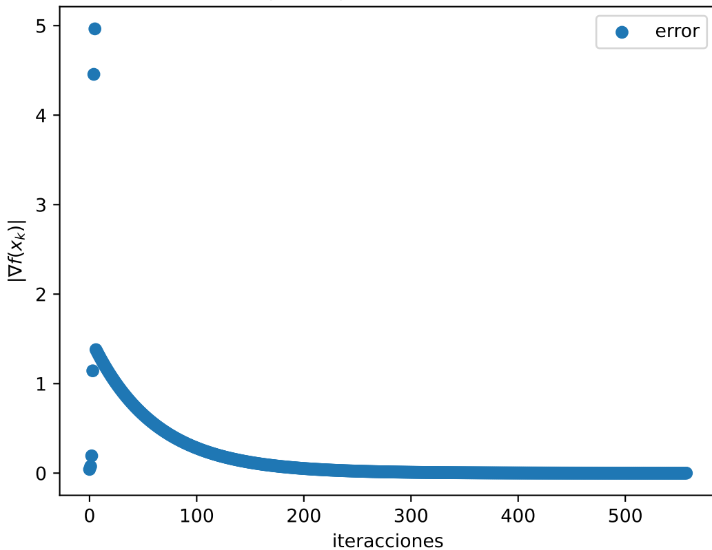
Gráfica |\nabla f(x_k)| de Hartmann \delta = 10.0
