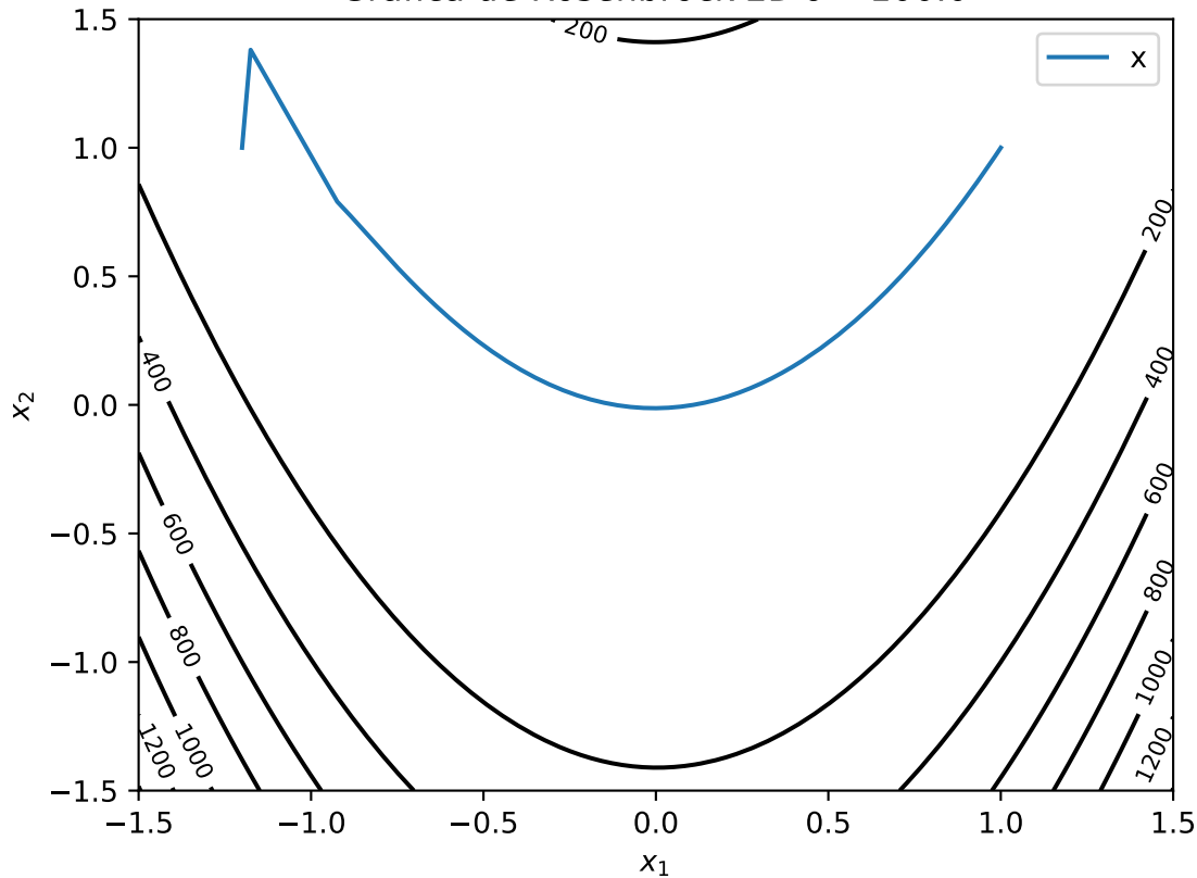
Gráfica de Rosenbrock 2D \delta = 100.0
