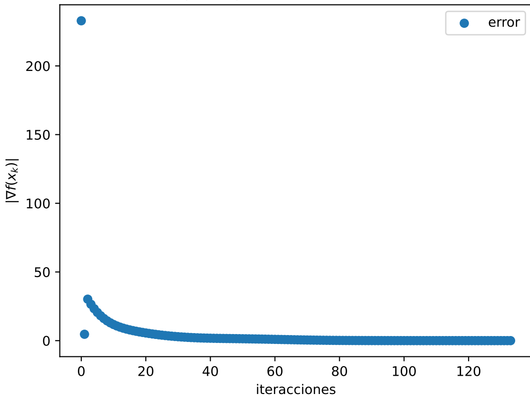
Gráfica |\nabla f(x_k)| de Rosenbrock 2D \delta = 100.0
