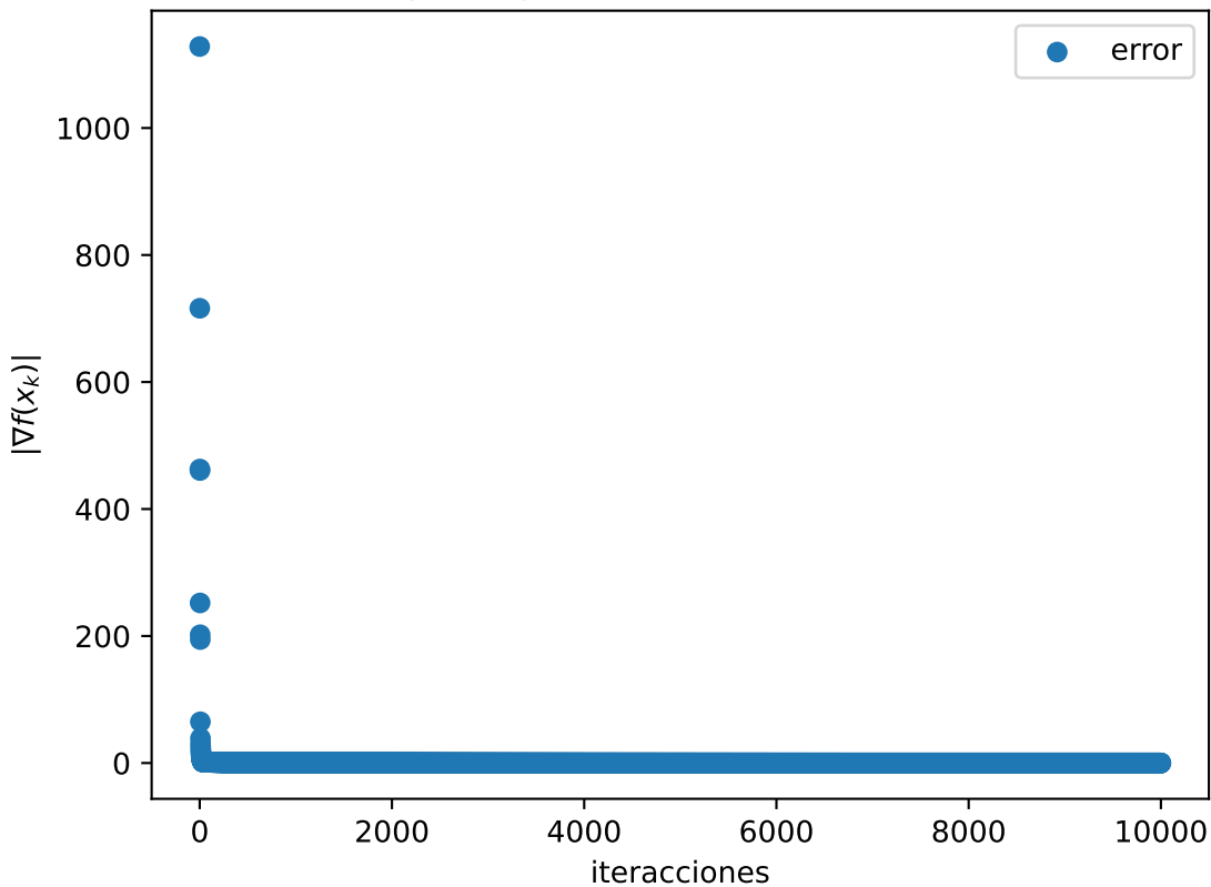
Gráfica |\nabla f(x_k)| de Rosenbrock 600D \delta = 100.0
