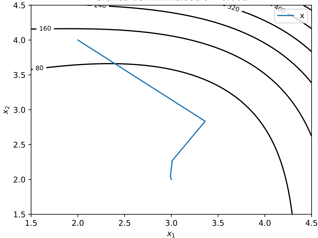
Gráfica de Himmelbau \delta = 0.001
