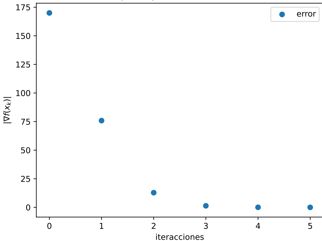
Gráfica |\nabla f(x_k)| de Himmelbau \delta = 0.001
