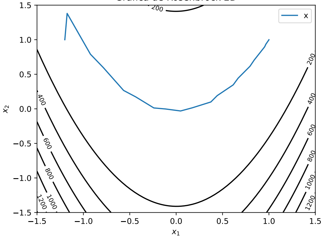
Gráfica de Rosenbrock 2D
