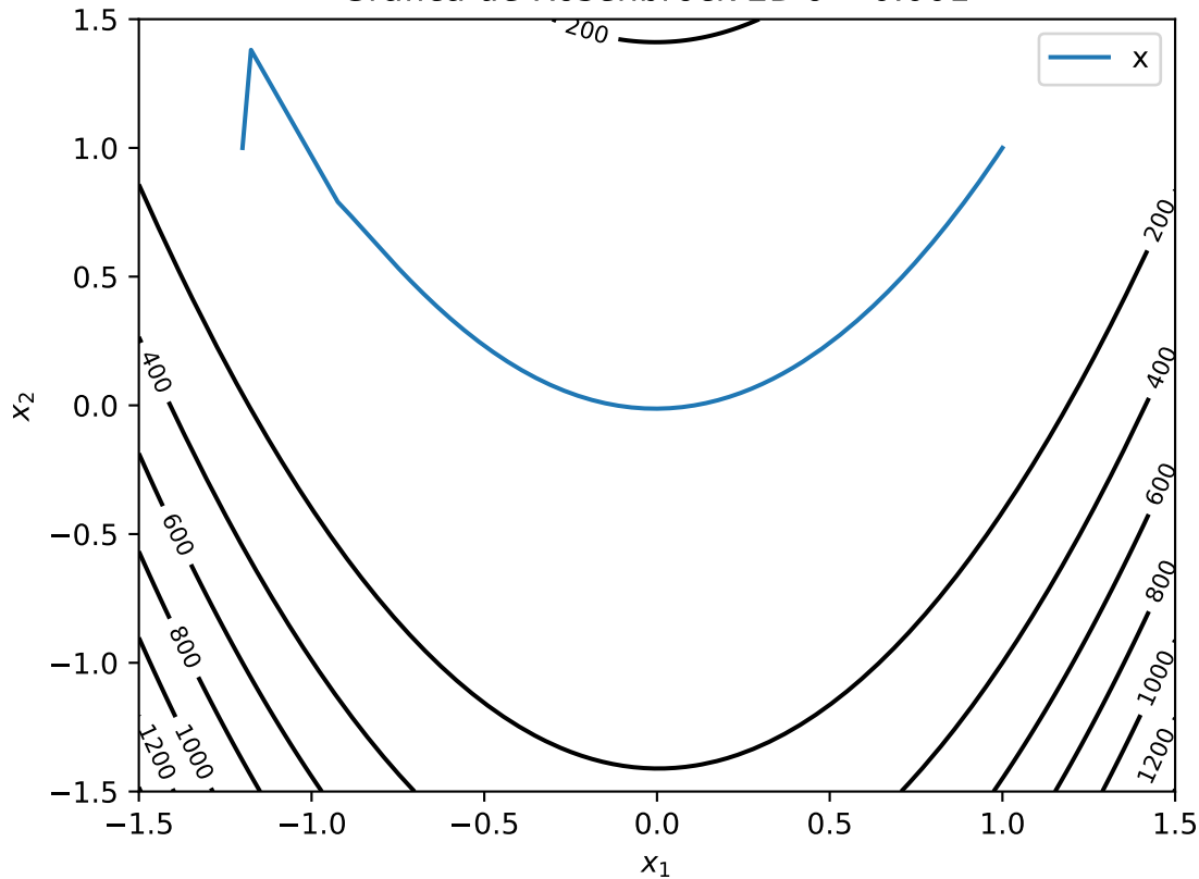
Gráfica de Rosenbrock 2D \delta = 0.001
