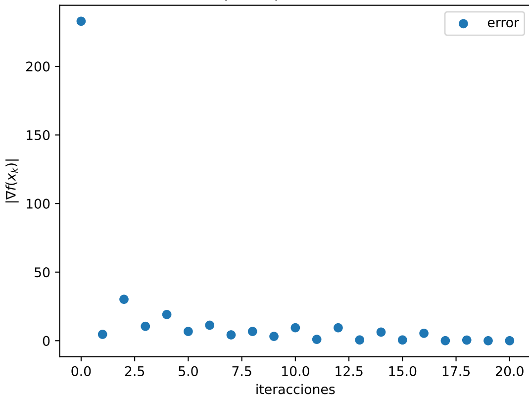
Gráfica |\nabla f(x_k)| de Rosenbrock 2D
