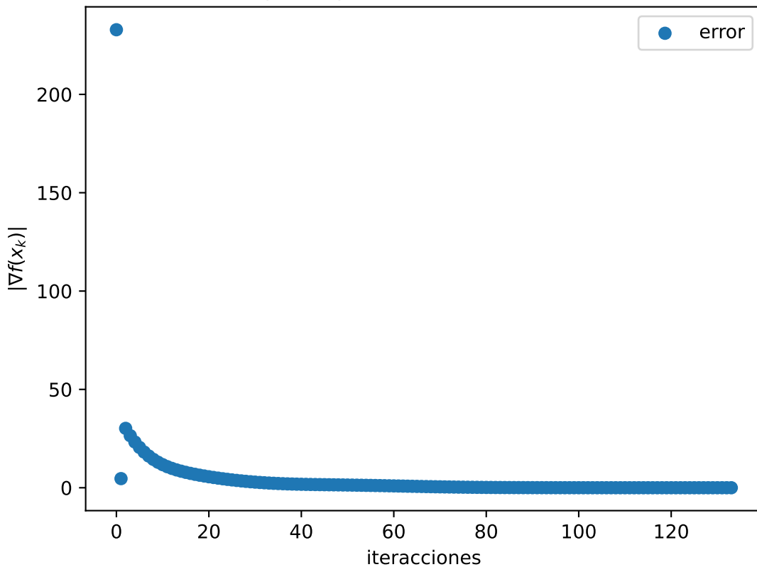
Gráfica |\nabla f(x_k)| de Rosenbrock 2D \delta = 0.001
