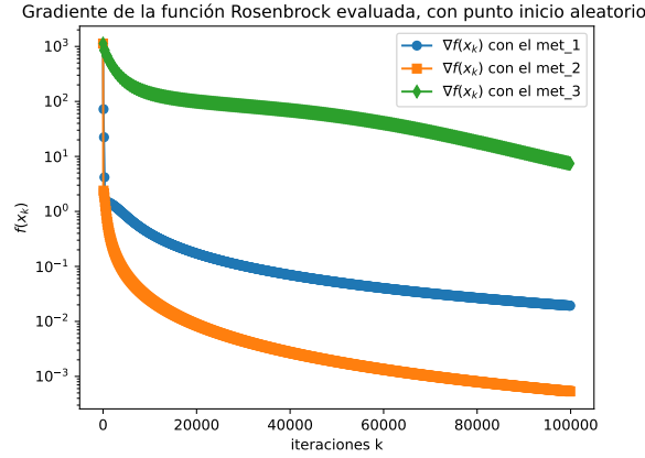
Figura 2.4: Gradiante de la función Rosenbrock evaluada, con punto inicio aleatorio
