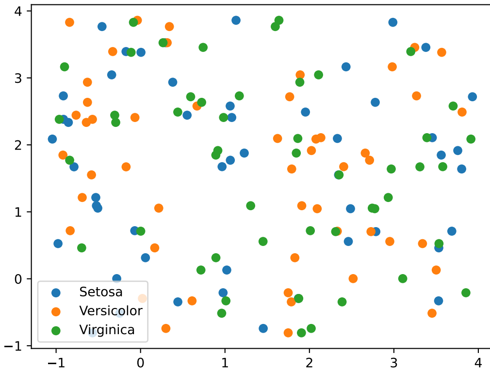
Escalado multidimensional \mathbb{R}^2 con aprox. \alpha de tipo 3
