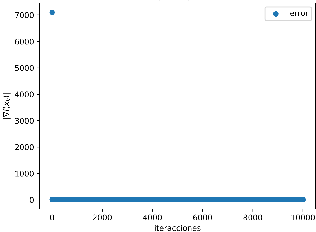
Gráfica |\nabla f(x_k)| de beale
