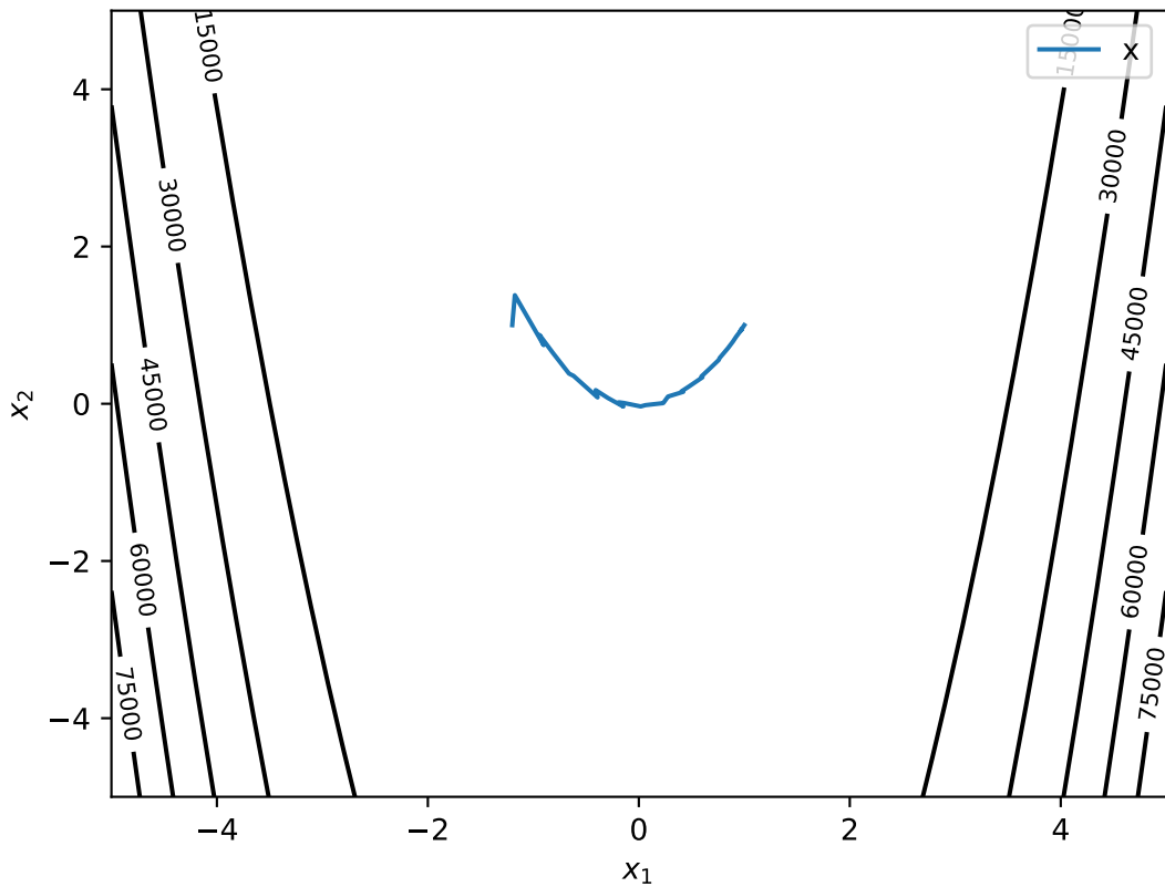
Gráfica de Rosenbrock
