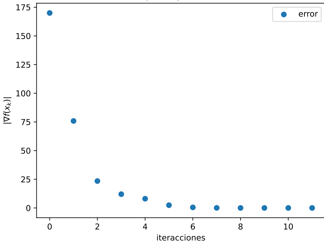
Gráfica |\nabla f(x_k)| de Himmelbau
