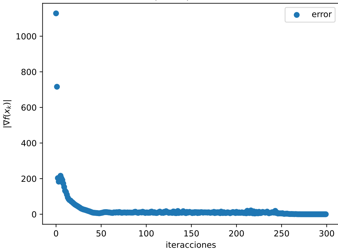
Gráfica |\nabla f(x_k)| de Rosenbrock
