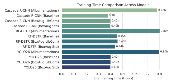
Figura 14: Comparación del tiempo total de entrenamiento por configuración.
