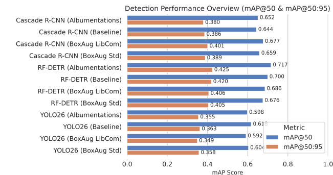
Figura 5: Panorama de mAP@0.5 y mAP@0.5:0.95 por configuración modelo-aumento, confirmando el orden RF-DETR, Cascade R-CNN, YOLO26 en ambas métricas.
