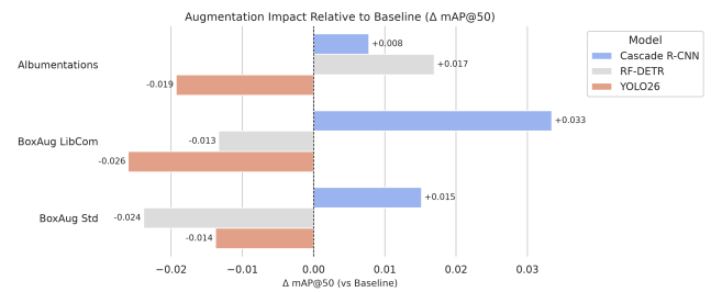
Figura 6: Impacto de las estrategias de augmentación respecto al baseline ( \Delta mAP@0.5).
