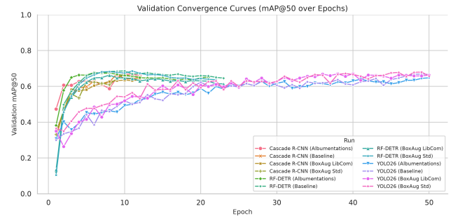
Figura 12: Curvas de convergencia de mAP@0.5 en validación durante el entrenamiento.
