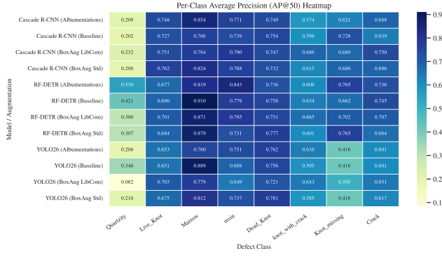
Figura 7: Mapa de calor de precisión promedio por clase de defecto (AP@0.5).
