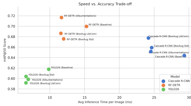
Figura 10: Compromiso entre velocidad de inferencia (ms/imagen) y precisión (mAP@0.5).
