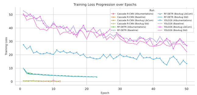
Figura 13: Progresión de la pérdida de entrenamiento por época para las 12 configuraciones.
