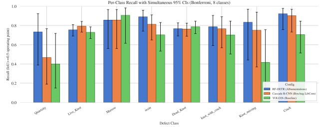
Figura 9: Recall por clase con intervalos de confianza simultáneos del 95% a nivel familiar para la mejor configuración de cada paradigma. Las barras de error son intervalos de Wilson al 99.375% por clase, es decir cobertura simultánea del 95% a nivel familiar sobre las 8 clases (Bonferroni).
