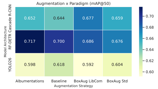
Figura 3: Matriz de rendimiento mAP@0.5 intersecando tres paradigmas de detección con cuatro estrategias de aumento.
