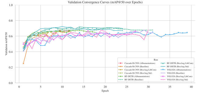
Figura 7: Curvas de convergencia de mAP@0.5 en validación durante el entrenamiento.
