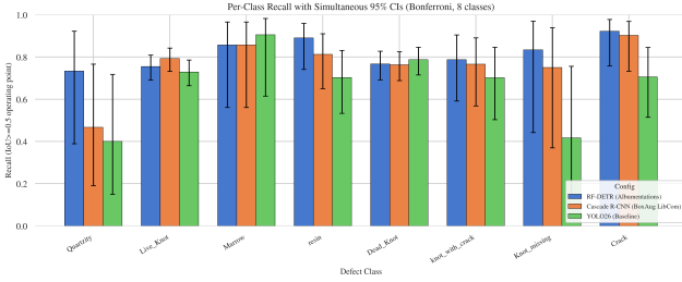
Figura 10: Recall por clase con intervalos de confianza simultáneos del 95% a nivel familiar para la mejor configuración de cada paradigma. Las barras de error son intervalos de Wilson al 99.375% por clase, es decir cobertura simultánea del 95% a nivel familiar sobre las 8 clases (Bonferroni).
