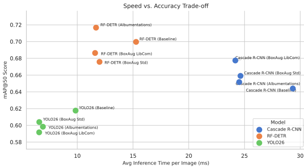
Figura 11: Compromiso entre velocidad de inferencia (ms/imagen) y precisión (mAP@0.5).
