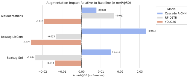
Figura 7: Impacto de las estrategias de augmentación respecto al baseline ( \Delta mAP@0.5).
