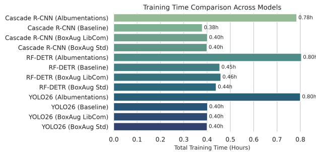
Figura 15: Comparación del tiempo total de entrenamiento por configuración.
