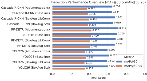
Figura 6: Panorama de mAP@0.5 y mAP@0.5:0.95 por configuración modelo-aumento, confirmando el orden RF-DETR, Cascade R-CNN, YOLO26 en ambas métricas.
