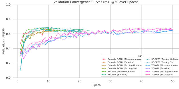
Figura 13: Curvas de convergencia de mAP@0.5 en validación durante el entrenamiento.
