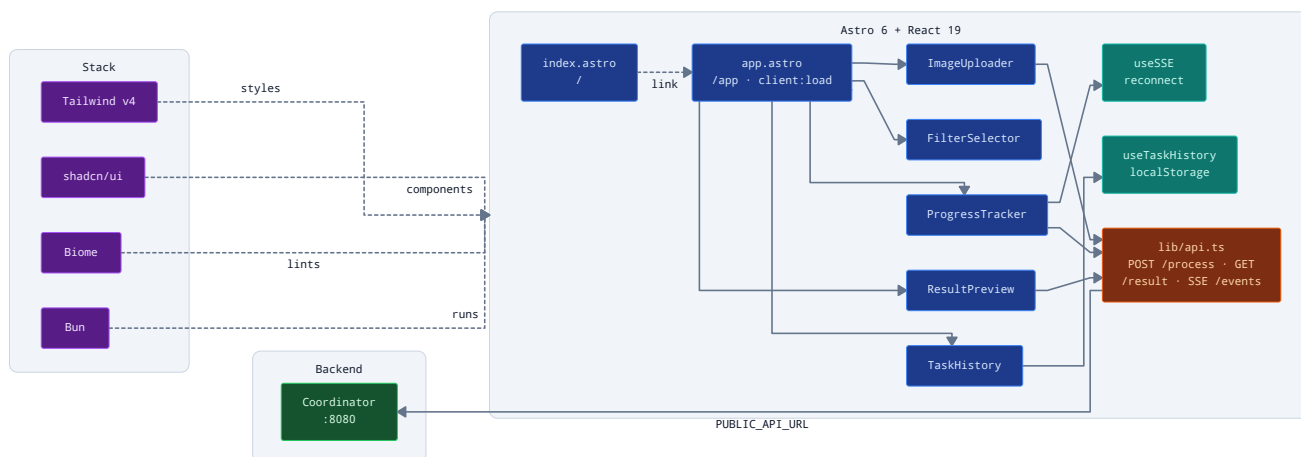
Figura 3. Diagrama de Componentes del Frontend de Microphoto
